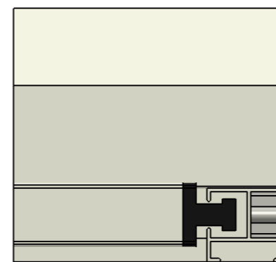
Onderaanzicht
